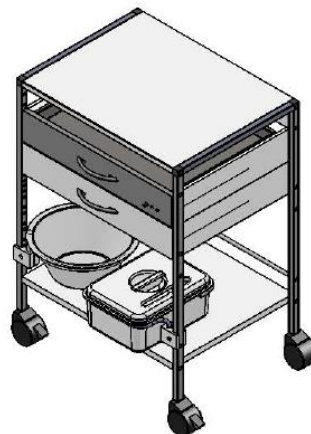
VARIOCAR® 60 GYNE 05355 600x450x830mm (L x S x K)
