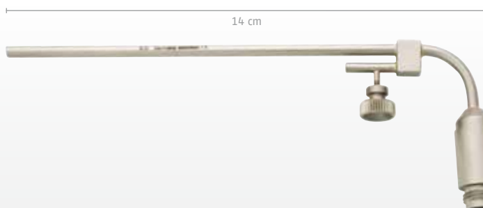
Fiberglas-Lichtträger für starre und spreizbare Laryngoskope, 14 cm Fiberglass lightcarrier for rigid and spreadable laryngoscopes, 14 cm
