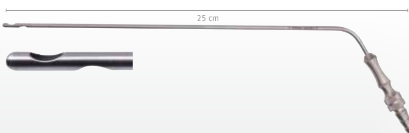
Saugrohr mit Unterbrecher, Spitze geschlossen, zwei seitliche Öffnungen 3,0 mm, 25 cm Suction tube with interruptor, tip closed, two side openings of 3.0 mm, 25 cm
