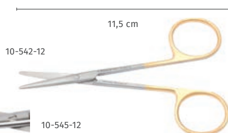
Schere, Hartmetall, stumpf-stumpf, 11,5 cm Scissors, tungsten carbide, blunt, 11.5 cm
