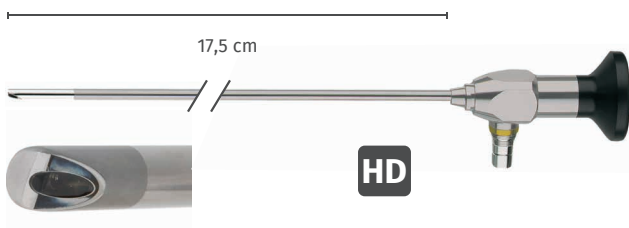
Laryngoskop, HD, autoklavierbar, 17,5 cm
