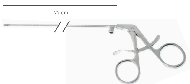
Laryngoskopie-Nadelhalter mit Spülkanal, mit Sperre, konischer Schaft (2,0 - 3,0 mm), 22 cm Laryngeal needle-holder with irrigation channel, with ratchet, conical shaft (2.0 - 3.0 mm), 22 cm 50-650-23
