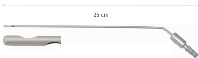
Saugrohr mit Unterbrecher, Spitze geschlossen, zwei seitliche Öffnungen 3,0 mm, 25 cm Suction tube with interruptor, tip closed, two side openings 3.0 mm, 25 cm
